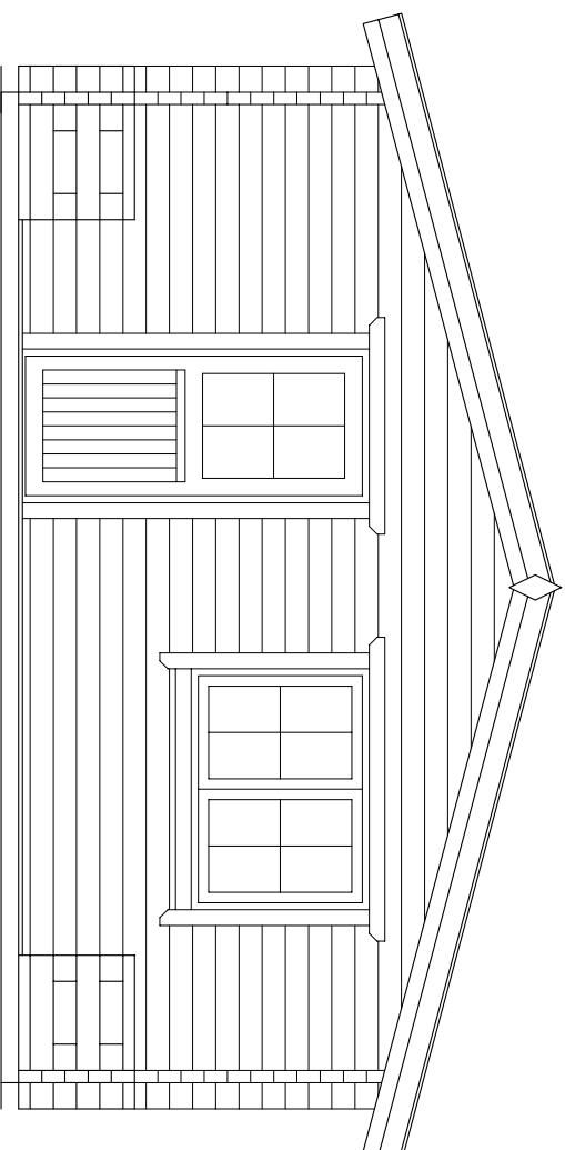
Ansicht-A
