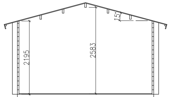
Qurschnitt A-A
