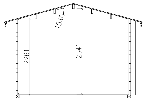
Querschnitt A-A
