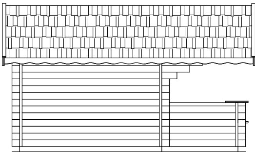
Ansicht -C
