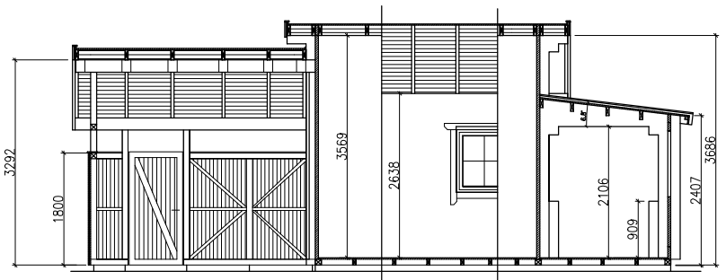
Querschnitt 1-1
