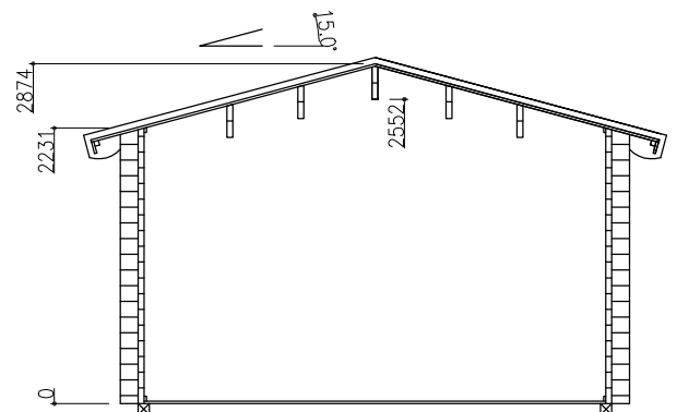
Querschnitt 1-1
