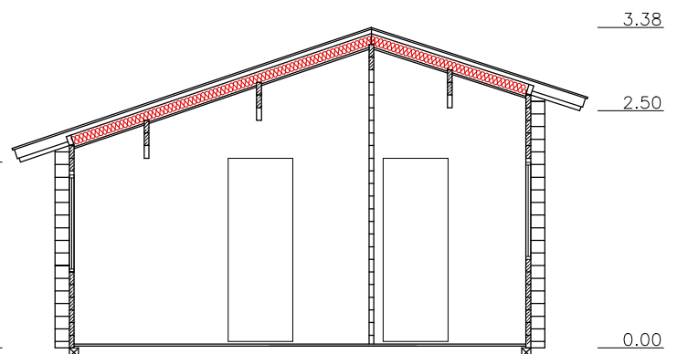
Schnitt A-A
