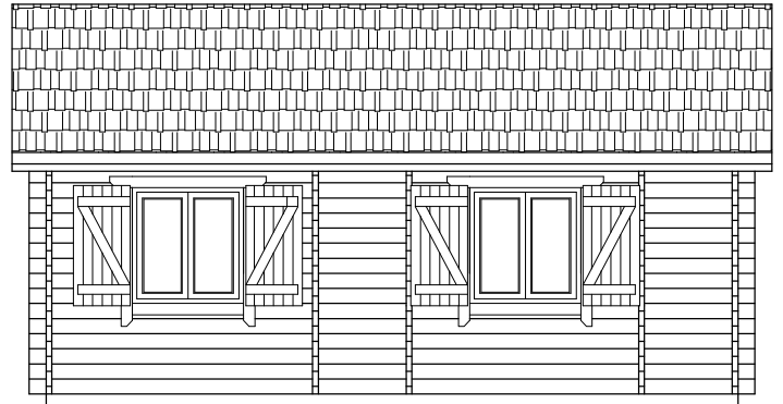
Ansicht -C
