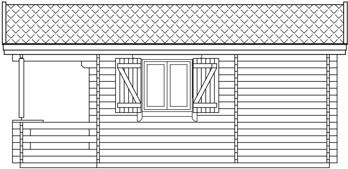
Ansicht -D
