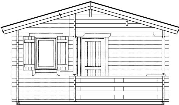
Ansicht -A
