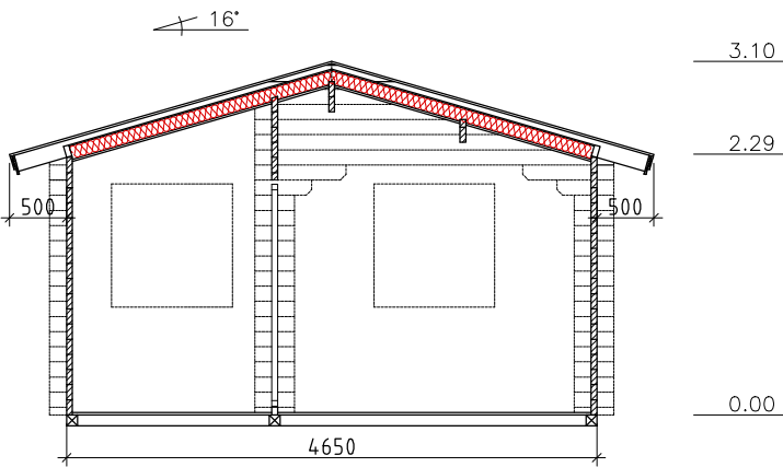
Schnitt A-A
