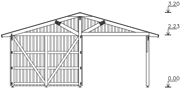
QUERSCHNITT -A
