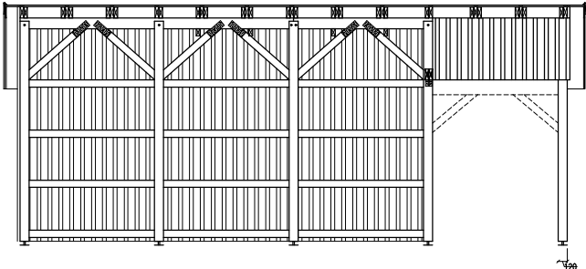
QUERSCHNITT -C
