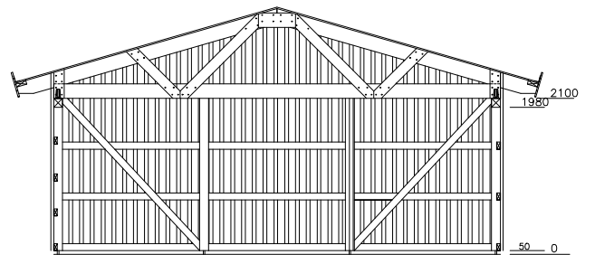
QUERSCHNITT - B
