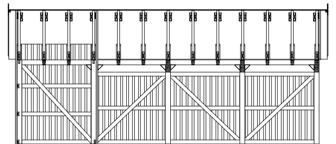
QUERSCHNITT - B
