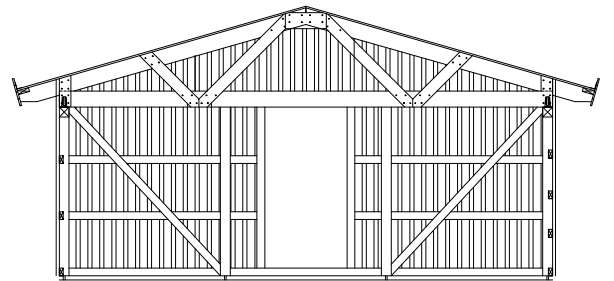
QUERSCHNITT - A
