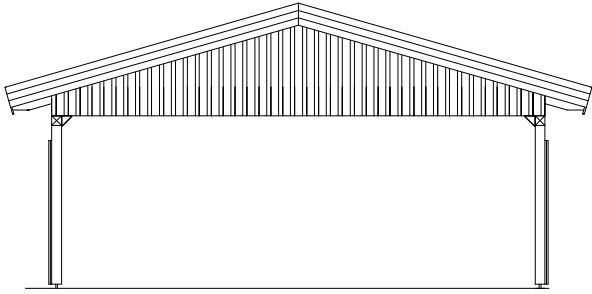
Ansicht - A
