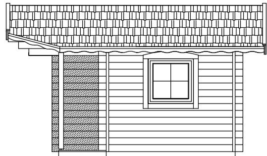
Ansicht -D
