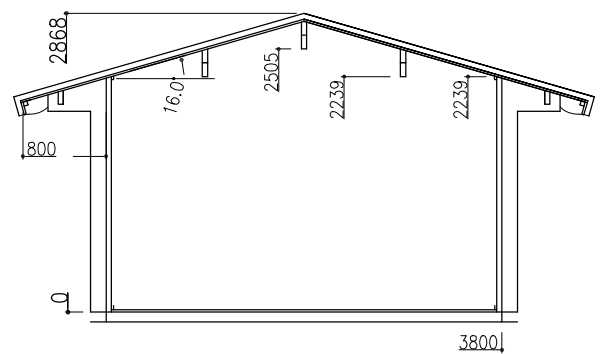
Querschnitt 1-1
