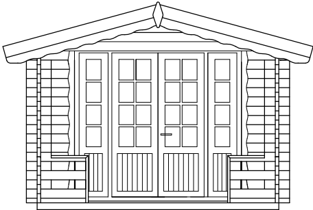
Ansicht -A
