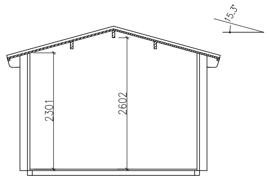
Querschnitt 1-1
